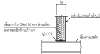
ลักษณะการติดตั้งบนพื้น/คานเหล็ก
