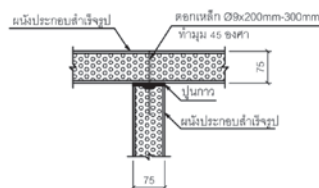
ลักษณะการต่อ "T"
