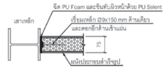
ลักษณะการติดตั้งกับเสาเหล็ก
