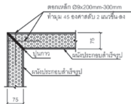
ลักษณะการต่อ "มุม 45 องศา"
