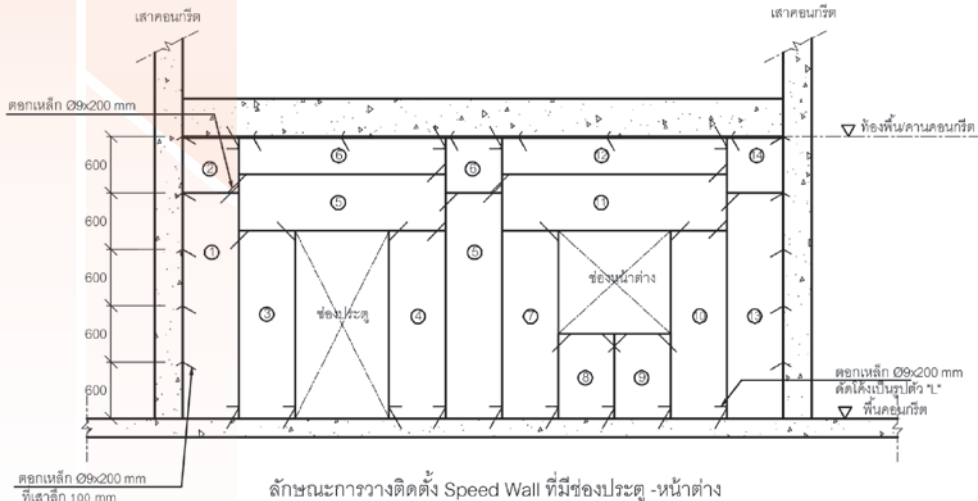
ขนาด, รูปแบบการใช้งานผนังประกอบสำเร็จรูป
