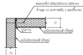
ลักษณะการต่อ "มุม 90 องศา"
