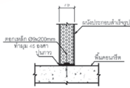
ลักษณะการติดตั้งบนพื้นคอนกรีต
